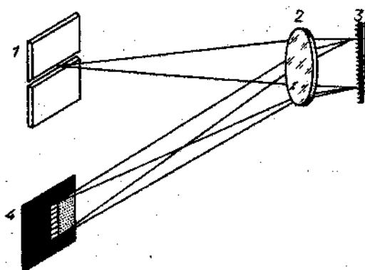
Рис. 14. Схема автоколлимационного спектрографа: 1 — щель; 2 — объектив, служащий коллиматором и камерой; 3 — дифракционная решетка; 4 — фокальная плоскость, в которой строится спектр
