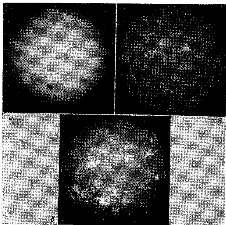
I. Вид диска Солнца в белом свете (a), в линии водорода H_{\alpha} (б), в линии К ионизованного кальция (в)
