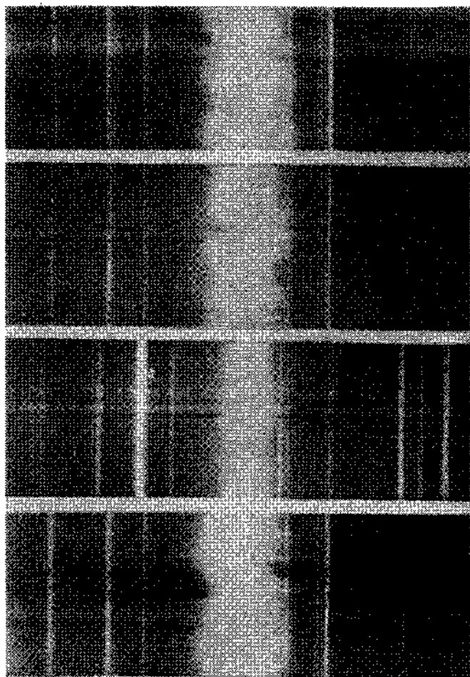
ХП. Вверху — спектр протуберанца в области линии H_\alpha (негатив). Более слабые линии, непрерывный спектр и линии поглощения, принадлежат рассеянному свету неба. Темная (на самом деле яркая) эмиссия — излучение протуберанца в линии H_\alpha , смещенная по спектру в синюю сторону от линии поглощения H_\alpha из-за движения с большой скоростью от Солнца к наблюдателю (эффект Доплера). Внизу — усы в линиях водорода H_\alpha (спектры 1-й, 2-й и 4-й сверху) и H_\beta (3-й спектр) (негатив)
