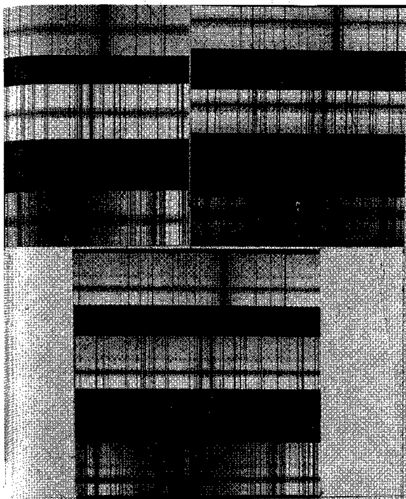
IX. Спектры трех пятен в области H (верхний спектр на каждой фотографии), в зеленой части спектра ( \lambda = 4920 \text{ \AA} ) (спектр в середине) и в области линии K (нижний спектр) (позитив)
